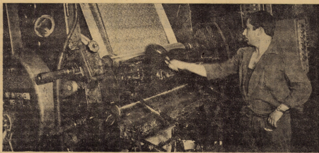
Întreprinderea „Tirnavă” Mediaș, secția finisaj. Modele de mare varietate și de creație proprie sînt aplicate țesăturilor cu ajutorul unor utilaje complexe — mașinile de imprimat în 6 culori Foto: Fred NUSS
