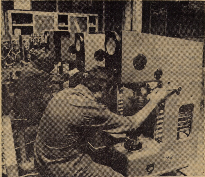
Operația de reglaj fin la un lot de aparate de încercat duritatea materialelor, tip BRINELL, în atelierul de mecanică fină a întreprinderii „Balanța” Sibiu Foto: Fred NUSS
