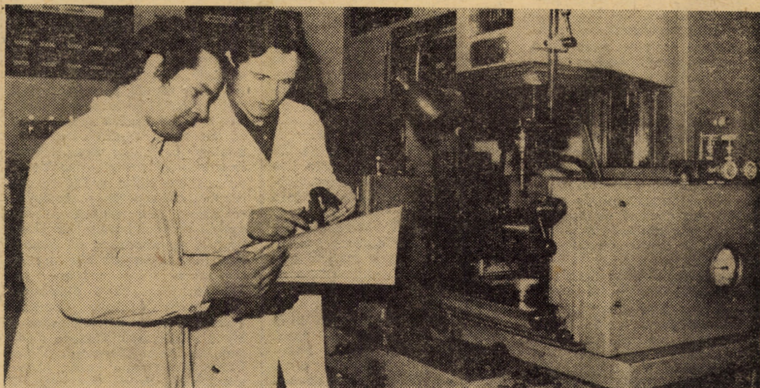
În laboratoarele modern utilizate ale Facultății de mecanică Sibiu, o mașină pentru prelucrări prin eroziune electrică permite executarea — în laboratorul de tehnica materialelor — a unor lucrări de mare complexitate
