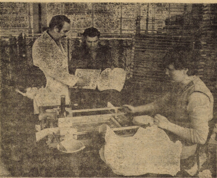
Ing. Eugen Jimon și maistrul de schimb Stelian Mănică verificînd calitatea decalcomaniilor în atelierul de imprimare al întreprinderii „Emailul roșu” Mediaș. Foto: Fred NUSS
