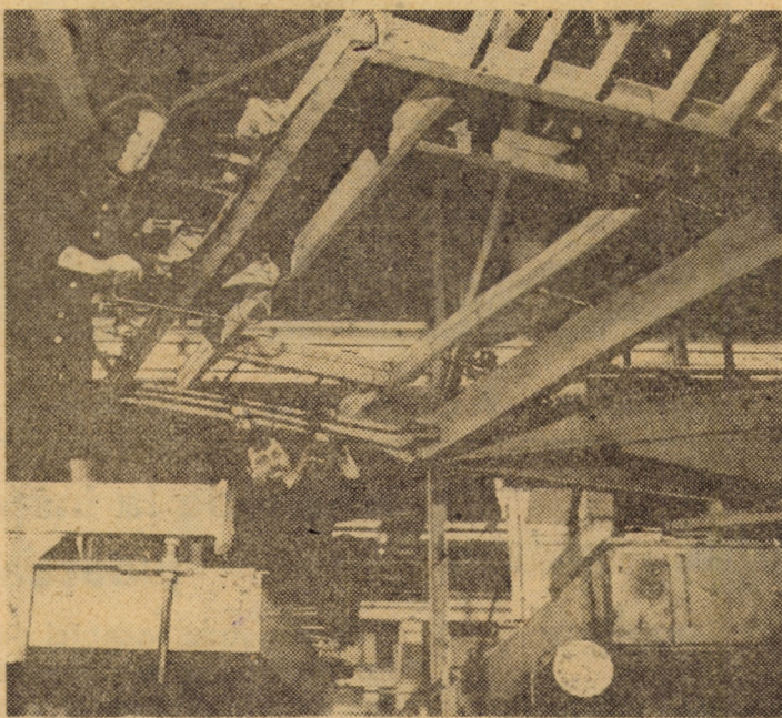
Întreprinderea mecanică Sibiu. Se montează noi agregate de termofomare cu patru posturi, destinat formării de piese din material plastic din semifabricate sub formă de plăci, folosite la fabricarea frigiderelor, în industria alimentară și a ambalajelor — utilaje realizate la înalți parametri în cadrul întrecerii socialiste.
