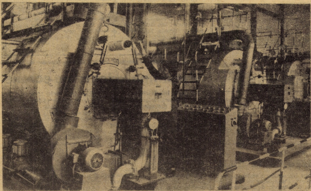
La centrala termică a întreprinderii „Steaua roșie” Sibiu există o preocupare constantă pentru reducerea consumului de gaz metan. În acest scop au fost realizate două instalații de recuperare a căldurii gazelor arse de la coș, obținându-se o creștere a temperaturii amestecului gazos în camera de ardere. Specialiștii intenționează ca în curând să îmbunătățească acest sistem de recuperare
