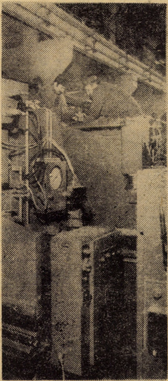
Întreprinderea mecanica Sibiu, secția montaj. În imagine lucrări de finisare la unul din produsele de bază și de serie mare, destinate exportului: Presă de indoit tablă de 100 tone-forță
