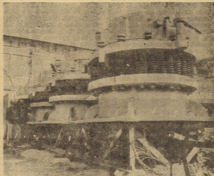
Dintre produsele de mare gabarit ale întreprinderii „Independența” Sibiu, destinate exportului, vă prezentăm — în imagine — un lot de consoare Ø 1250 mm, gata pentru a fi expediate beneficiarilor Foto: Fred NUSS
