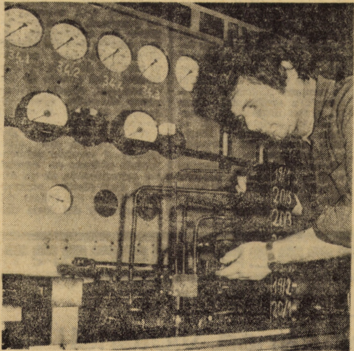
Unul din modernele standuri de probă pentru aparatură de 315 bari, realizat prin autodotare de specialiștii Fabricii de elemente hidropneumatice a întreprinderii „Balanța” din Sibiu
