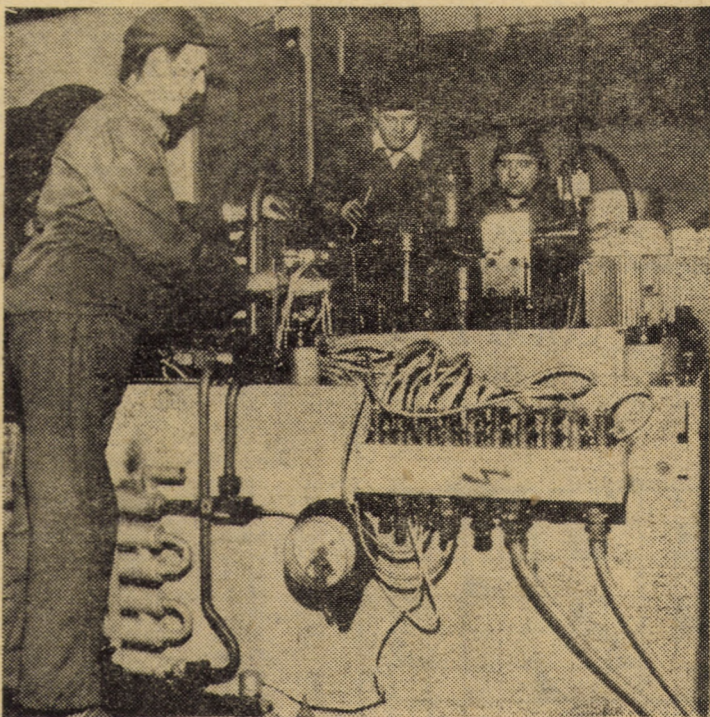
Recent, la întreprinderea „Mecanica” Sibiu a fost realizată în premieră o presă de decupaj fin de 400 tone, aflată în prezent în probe tehnologice. Noul utilaj de mare complexitate permite decuparea pieselor fără a mai fi nevoie de o finisare ulterioară a acestora. În fotografie: comuniștii Nicolae Cerciu, șef de echipă, Ioan Rădoi și Mihai Seiler, lăcătuși, lucrînd la finisarea utilajului care va fi expedit beneficiarului pînă la finele acestui an. Foto: Fred NUSS
