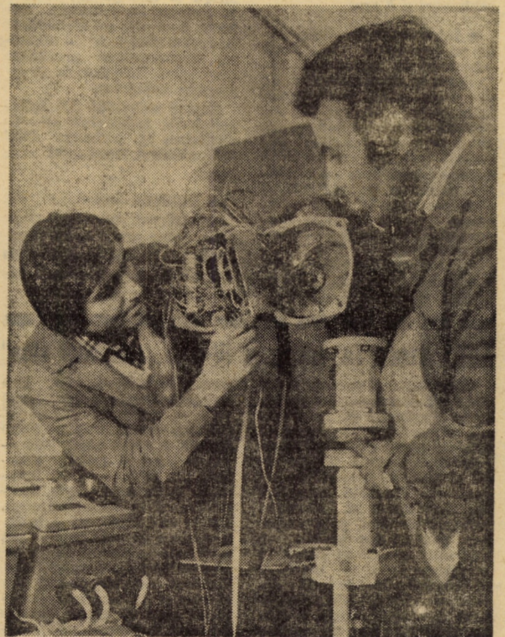
Probe de fiabilitate în atelierul de prototipuri al ICEMENERG, filiala Sibiu, la un servomotor electric cu acționare prin roțire destinat unor instalații electrice. În imagine sing. Aurel Mihăilescu și sing. Gheorghe Bărbat, efectuînd probele la stand Foto: Fred NUSS
