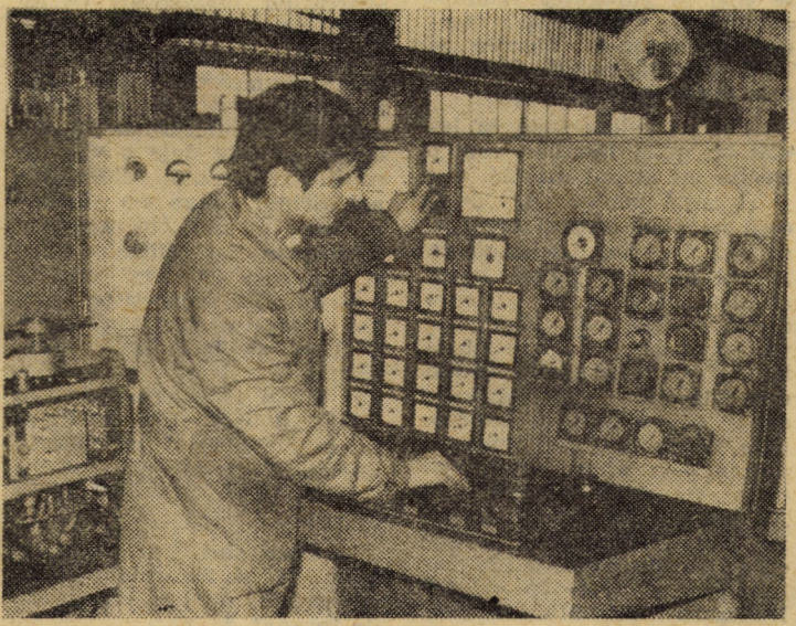
În imagine un stand de probă pentru aparatură hidropneumatică realizat prin autoutilare de către specialiștii Fabricii de elemente hidropneumatice a întreprinderii „Balanța” Sibiu. Foto: Fred NUSS
