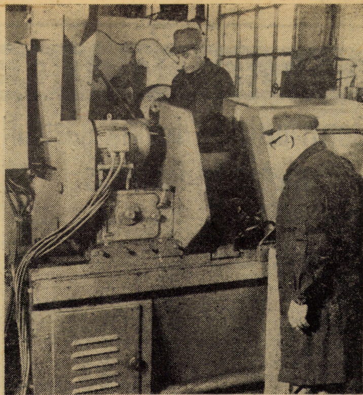
Recent specialiștii secțiilor mecanică II și III, în colaborare cu atelierul 7 de proiectare ale întreprinderii „Independența” Sibiu, au conceput și realizat o mașină automată de strunjit bolțuri la ambele capete. Astfel de utilaje se importau pînă nu demult. Prin intrarea în funcțiune a acestui utilaj cu ciclu automat, productivitatea muncii la această operație a crescut cu 200 la sută, creîndu-se posibilitatea ca un muncitor să deservească mai multe mașini. De remarcat că noul produs a fost realizat integral cu elemente și subansamble produse în țară
