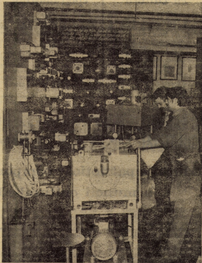
Vă prezentăm montajul panourilor hidropneumatice de înaltă complexitate la Fabrica de elemente hidropneumatice a întreprinderii „Balanța” Sibiu.
