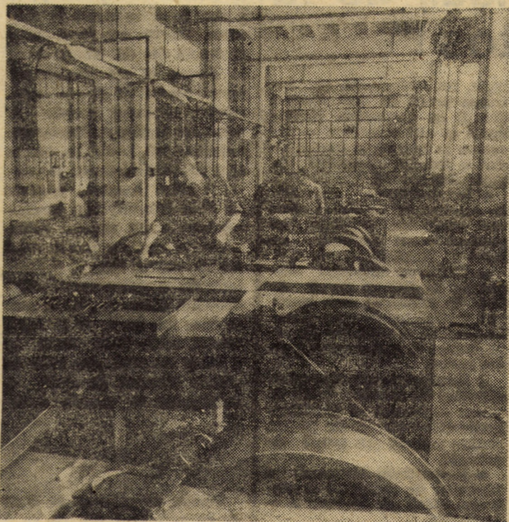
Întreprinderea „Flamura roșie” Sibiu, sectorul metal II. — Vă prezentăm moderna linie de laminare și prelucrare a sirmei în diferite profile, necesare pentru producția de accesorii textile Foto: Fred NUSS
