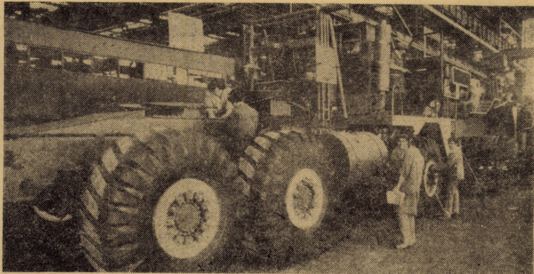
Întreprinderea mecanică Mirșa: aspecte de la linia de montaj a autovehiculelor pentru transport utilaj petrolier. Foto: Fred NUSS
