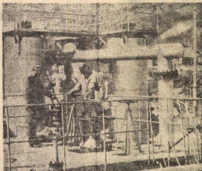
Imagine de la stația de uscare gaze Tăuni; efectuarea manevrelor pentru schimbarea ciclului de uscare a gazului metan
