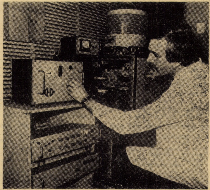
Printre dotările recente ale laboratorului pentru studiul metalelor al Facultății de mecanică Sibiu se inscrie și o instalație complexă de metalizare in vid (în fotografie). Astfel baza materială a acestui laborator se cifrează în prezent la cca 45 milioane lei, oferind largi posibilități de cercetare. Foto: Fred NUSS
