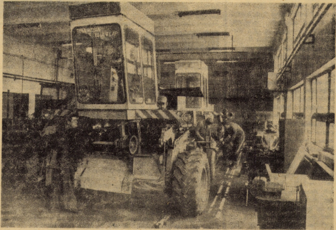
La noul sediu al Stațiunii pentru mecanizarea agriculturii din Ocna Sibiului — de unde vă redăm imaginea de față — se execută reparații capitale la utilaje agricole cum sint mașinile „WINDROVER” E 301 și E 302, provenite din județul Sibiu cit și din alte județe. Pe lângă atelierul de bază, aici mai funcționează o serie de ateliere anexă cum este cel de reparații electrice și de sudură, prelucrări mecanice, instalații hidraulice, un grup social, vestiare și o centrală termică, toate insumind o suprafață totală de peste 650 mp. Foto: Fred NUSS
