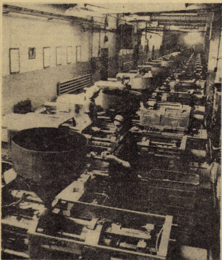
Vedere parțială a atelierului injectat mase plastice, aparținînd secției articole de scris de la binecunoscuta întreprindere „Flamura roșie” Sibiu Foto: Fred NUSS
