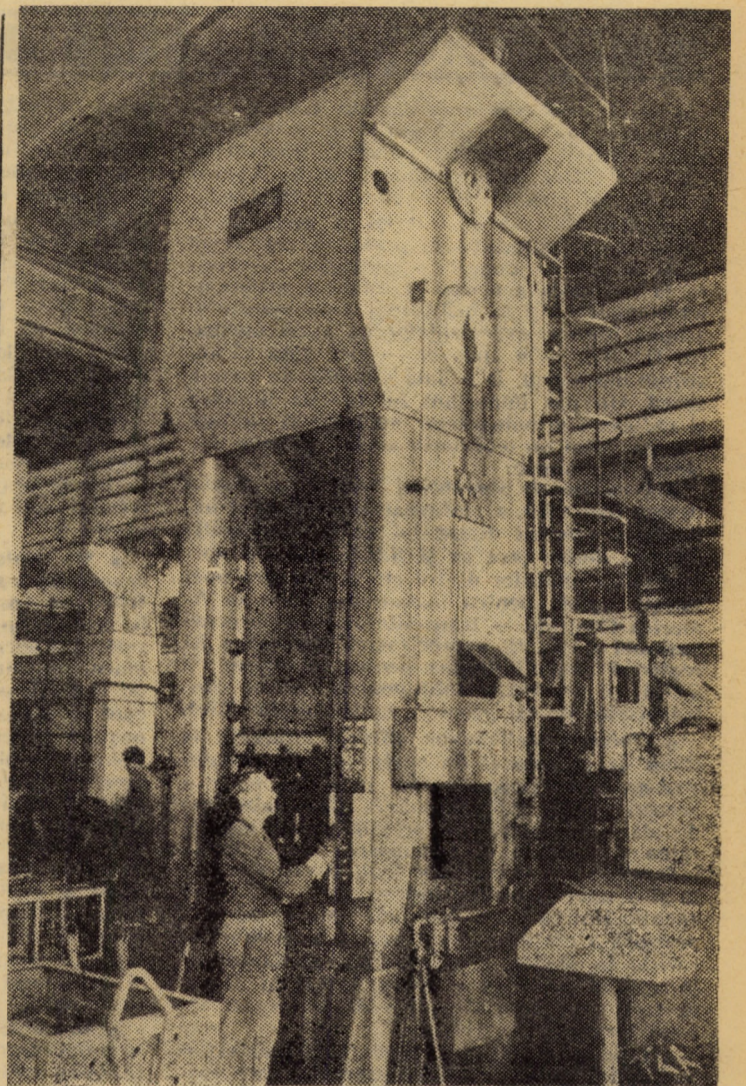
În atelierul debitare al I.M.A.I.A. Sibiu, la o presă de 400 tone - cel mai mare utilaj în cadrul unității - sint prelucrate piese cu pro- file complexe, necesare construcțiilor de utilaje agricole
