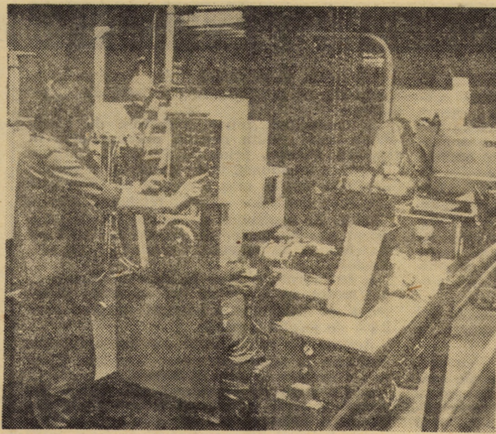
Linie modernă de prelucrat cruci cardanice la I.P.A. Sibiu. În prim plan: mașina de rectificat cu comandă program, utilaj de înaltă tehnicitate Foto: Fred NUSS
