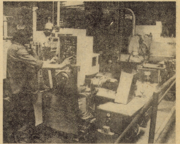
Întreprinderea „Balanța” Sibiu. Înainte de expediere la beneficiar, la standuri special amenajate se efectuează etalonarea balanțelor Foto: Fred NUSS
