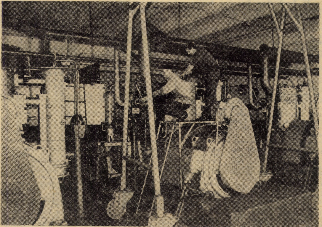
I.M.A.I.A. Sibiu. Aspect din moderna stație de compresoare care asigură aerul tehnologic necesar secțiilor de producție, întreținută exemplar de către mecanicii Francisc Babeș și Vasile Comănici. Colectivul oamenilor muncii din întreprindere, obține zi de zi însemnate realizări cu care întâmpină ziua de 23 August Foto: Fred NUSS
