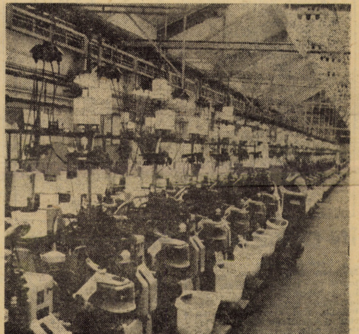
Vedere din hala mașinilor de tricrat a întreprinderii de ciorapi „7 Noiembrie”, Sibiu — una din numeroasele capacități de producție ridicate în cursul ultimilor 20 de ani în municipiul Sibiu Foto: Fred NUSS
