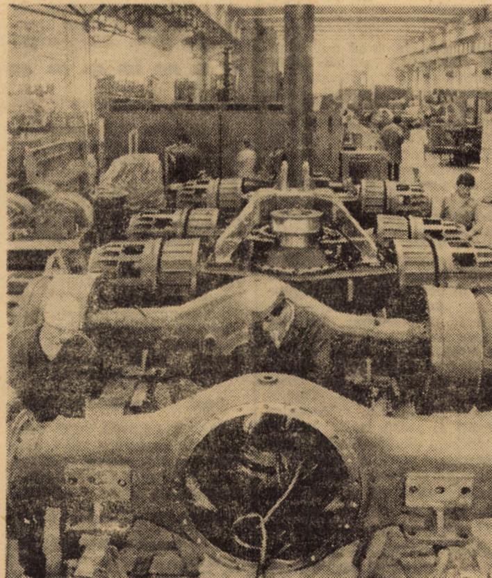
Întreprinderea mecanică Mirșa — Vedere parțială a liniei de montaj punți pentru autobasculantele de 55 t.f. Foto: Fred NUSS
