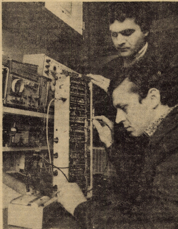
Secția electrificare, centralizare și telecomandă a Stației C.F.R. Sibiu. Vă prezentăm o secvență de lucru din Laboratorul de verificat și reparat sisteme de curenți purtători, ceasuri electronice și aparatul de telecomunicații. La masa de verificare: Florea Ungureanu și Simion Roșca, doi dintre tinerii electroniști cu o bună pregătire profesională care, prin munca lor de zi cu zi, contribuie la buna funcționare a întregului aparataj aferent instalațiilor de centralizare și telecomandă. Foto: Fred NUSS
