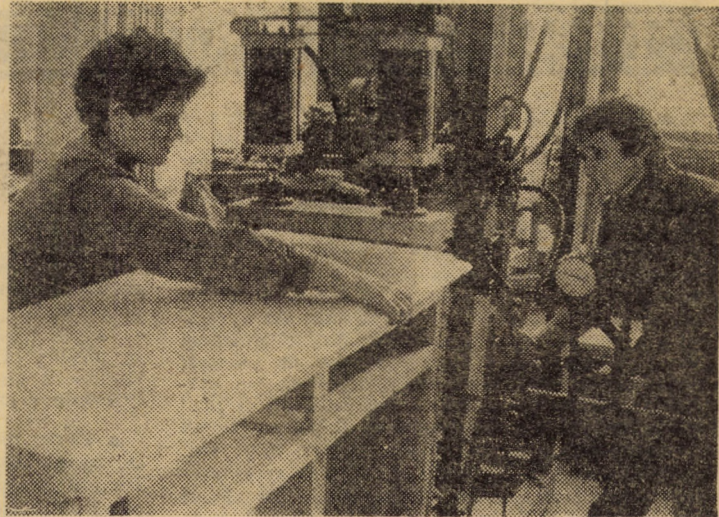
Fabrica de mobilă II, aparținând de I.P.L. Sibiu. Colectivul secției montaj a realizat, prin autofabricarea, un dispozitiv de asamblat cu acționare pneumatică, folosit cu bune rezultate la montarea diferitelor corpuri de mobilă Foto: Fred NUSS
