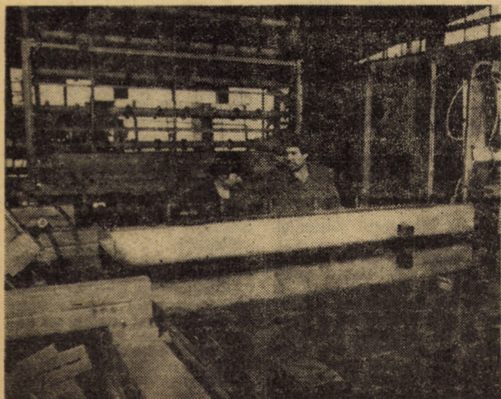
Întreprinderea de geamuri Medias. În imagine — instalația de tras geam pe orizontală Foto: Fred NUSS
