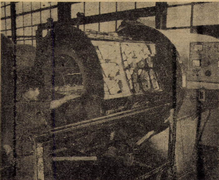
Întreprinderea de geamuri Medias: instalația pentru depunerea vaporilor de aluminiu în vid înaintat, pentru oglinzi retrovizoare Foto: Fred NUSS
