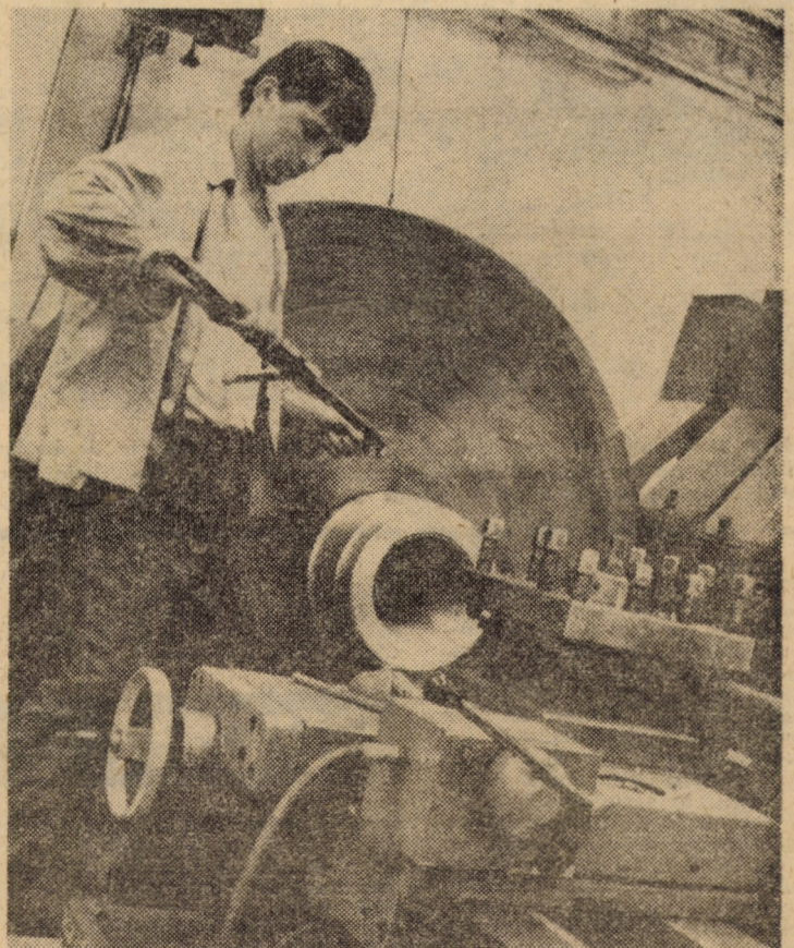
Prelucrarea prin așchiere a pieselor de mare gabarit în secția punți motoare a întreprinderii mecanice Mișsa Foto: Fr. NUSS
