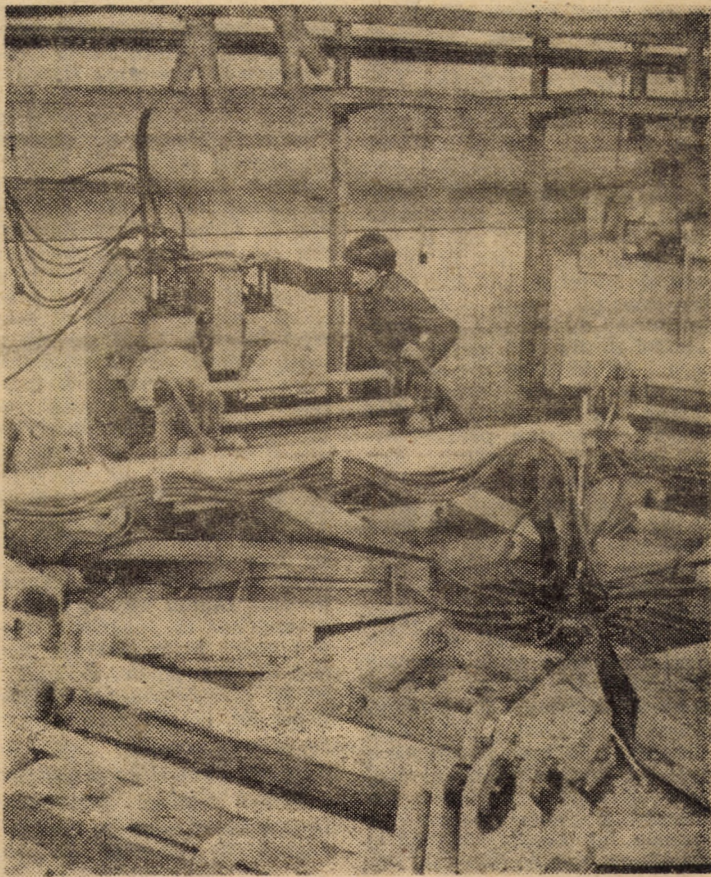
Vă prezentăm o vedere parțială din atelierul polizat automat al întreprinderii de cuțite Ocna Sibiului unde, printre alte utilaje de mare capacitate funcționează și agregatul de lustruit tacimuri (în fotografie), avînd o capacitate de 6000 produse într-un schimb. Pînă nu demult această operație era efectuată manual
