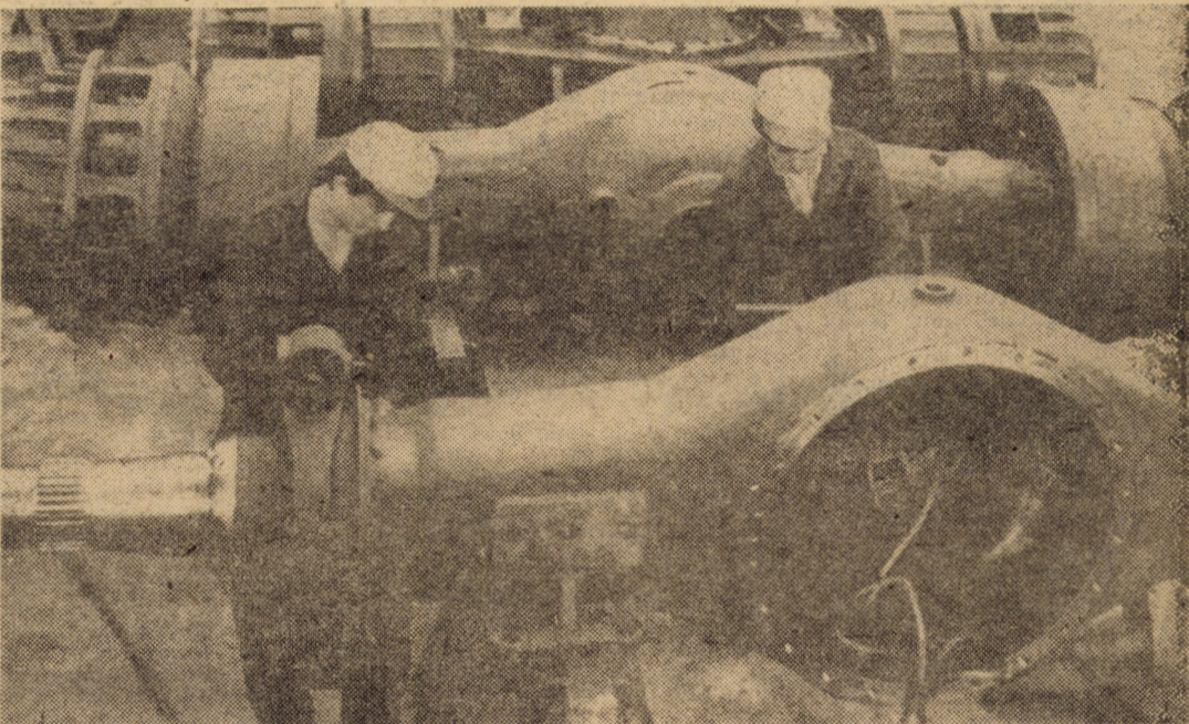
Imagine surprinsă la montajul punților motoare pentru autobasculante grele la întreprinderea mecanică Mirza. Foto: Fred NUSS
