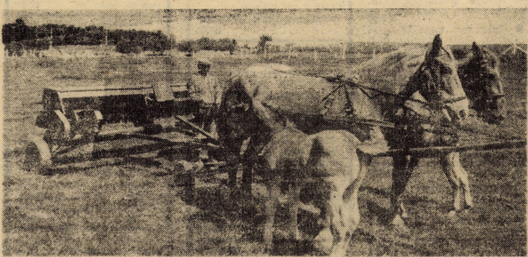
Vă prezentăm o mașină de aplicat îngrășăminte chimice pe pajști și suprainsămîntat, cu tracțiune hipo, realizată la Ferma de producție din Săliște a întreprinderii de îmbunătățiri și exploatare a pajștilor Sibiu. Utilajul a fost confecționat dintr-o mașină SUP-21 reformată, avînd lățimea de lucru de 2,5 metri și un randament de 2,5-4 ha/zi, funcție de pantele pe care se lucrează
