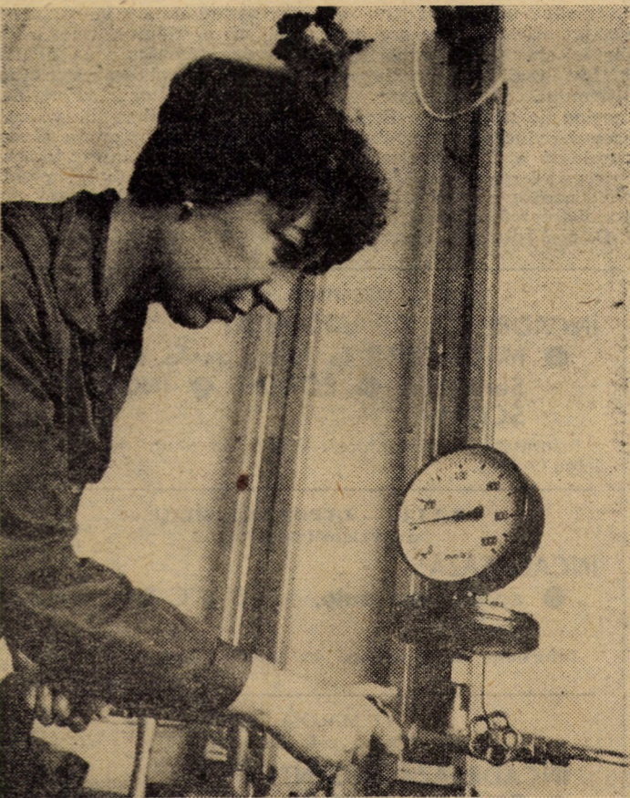
În laboratorul de metrologie al I.U.P.S. Sibiu, manometrele folosite la centrala termică, stația de oxigen, compresoare și alte utilaje din atelierele de producție ale unității, sînt supuse periodic unor verificări cu ajutorul unor instalații speciale, deservite de Susana Ciovică, verificator, A.M.C. Foto: Fred NUSS
