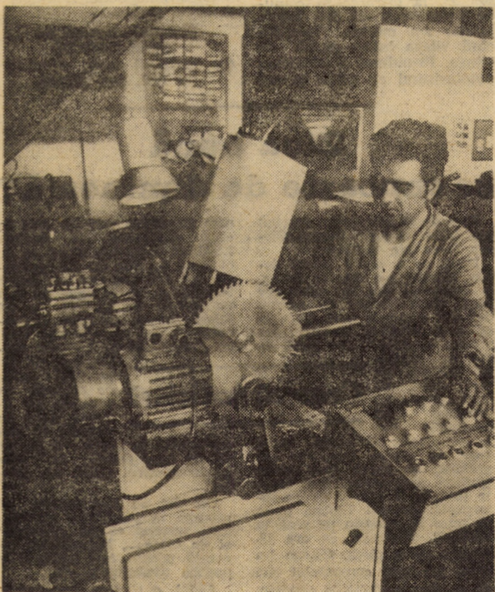
I.U.P.S. Sibiu: Un nou utilaj realizat în cadrul întreprinderii, prin autoutilare: mașina de ascuțit cu acționare hidraulică la care a contribuit, prin valoroase idei de concepție și șeful de echipă Ioan Nistor (în fotografie). Printre avantajele noii mașini pot fi enumerate: o mai mare precizie la prelucrare, siguranță, fiabilitate, creșterea productivității muncii cu 30 la sută și reducerea efortului valutar
