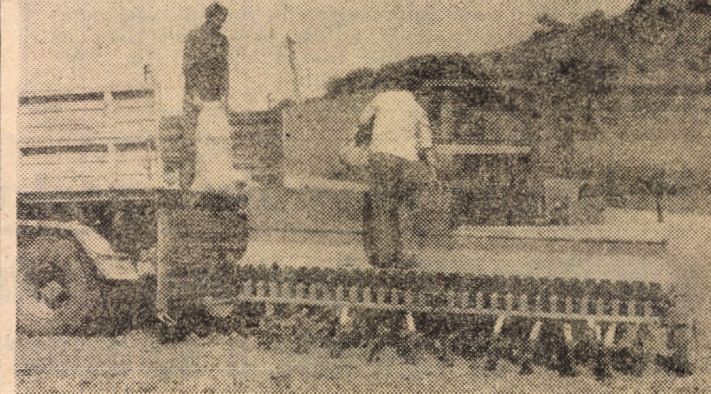
Mașina de semănat (mecanizator Teodor Prus, secția de mecanizare Blăjeștii de Jos) antrenată la semănatul orzului, cu tuburile lipsă
