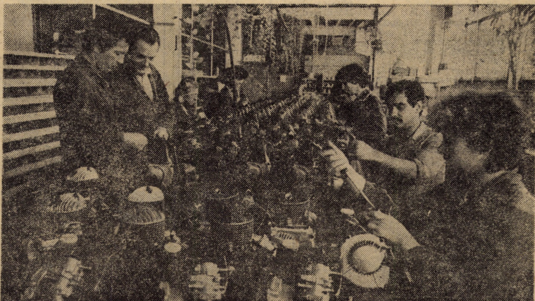
I.U.P.S. Sibiu. Prin înlocuirea unor componente metalice cu altele din masă plastică, motoferastrăile de tipul FM-75-5 de 4 C.P. prezintă acum o greutate mai redusă, scurindu-se totodată timpul de montaj al acestora
