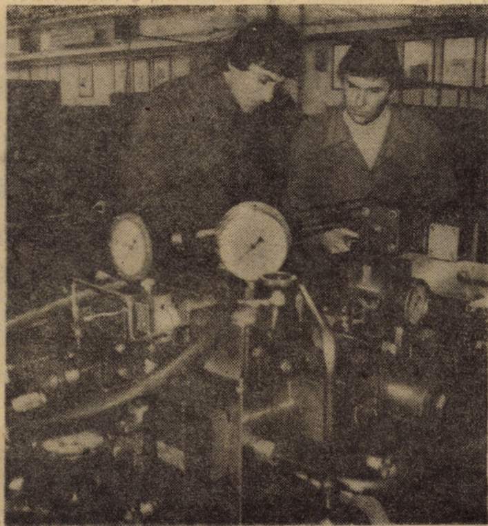
Fabrica de elemente hidropneumatice a întreprinderii „Balanța” Sibiu. Lăcătușul Vasile Bogdan și electricianul Cornel Bîanu verificînd presiunea pe circuite la un panou hidraulic pentru comanda mașinilor unelte Foto: Fred NUSS
