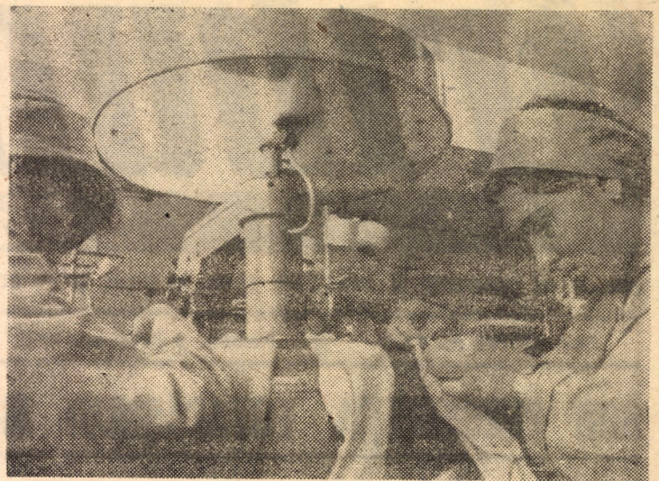
În atelierele bine utilitate ale Liceului textil „7 Noiembrie” din Sibiu, elevii ultimelor clase desfășoară practica productivă. În fotografie, un aspect de muncă de la mașinile de incheiat ciorapi
