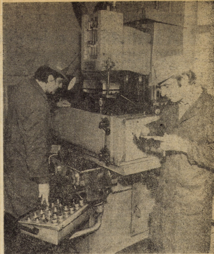
Compartimentul prelucrării prin electroeroziune — unul din locurile de muncă „cheie” al secției sculărie de la „Flaro” Sibiu, unde se realizează S.D.V.-uri de mare complexitate. Foto: Fred NUSS
