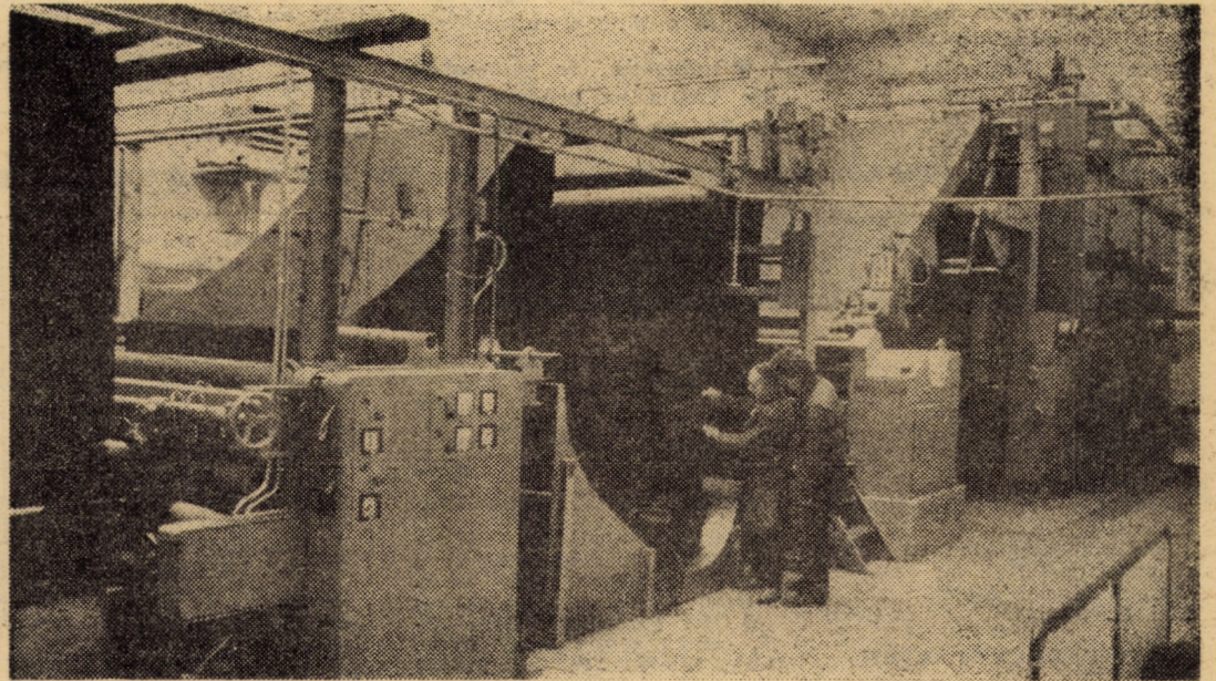
Imaginea de față prezintă un utilaj de mari proporții din secția finisaj a întreprinderii „Lăbertatea” din Sibiu: mașina de uscat și termofixat stoffe, avînd o capacitate de prelucrare de 13 000 mp stofă într-un schimb. La această mașină a fost montată o instalație de recuperare a căldurii, obținîndu-se astfel în 1986, o economie de energie electrică de 50 MWh și cea 1 000 mc gaz metan.
