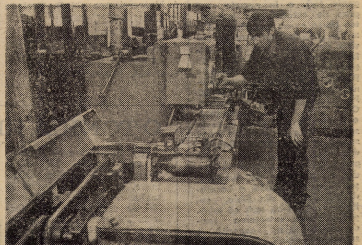
Vă redăm o secvență de muncă din atelierul prelucrării mecanice de la unitatea I – creioane, a I.P.L. Sibiu. În prim-plan: linia automată de confecționat creioane, asigurând 5 operații diferite de prelucrare Foto: Fred NUSS
