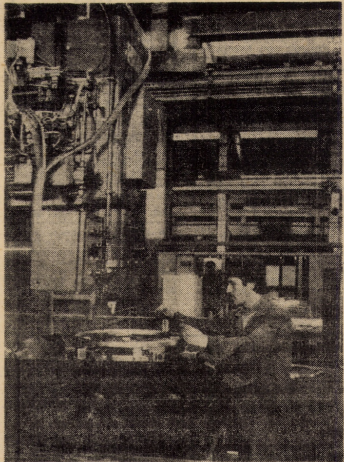
Întreprinderea mecanică Sibiu: în secția prelucrări mecanice, la o mașină CP2 dotată cu comandă numerică, comunistul Ioan Irod, frezor, execută lucrări de finisaj cu înaltă precizie
