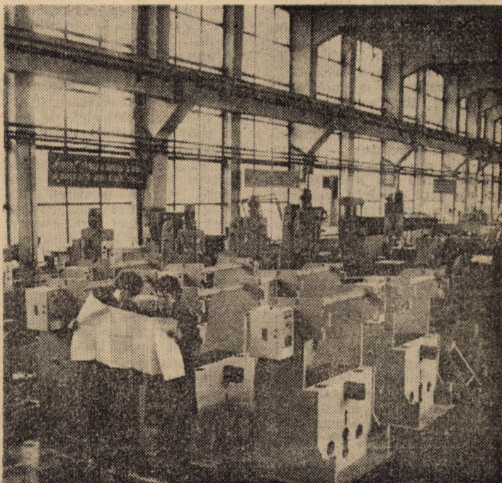
Vă redăm o vedere parțială din secția sculărie a întreprinderii mecanice Sibiu. În prim-planul fotografiei: un lot de prese de indoit tablă de 25 t.f., în faza de montaj Foto: Fred NUSS
