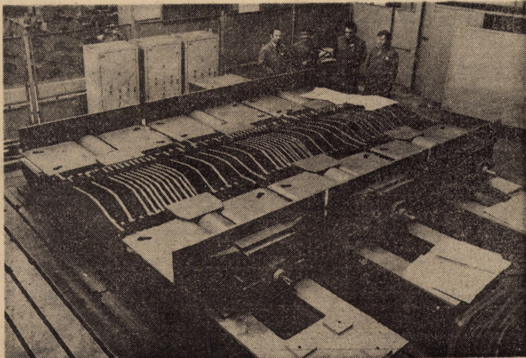
Rolgang la ferăstrău — una din componentele importante ale laminorului, livrate în avans de către colectivul de la „Independența” Sibiu
