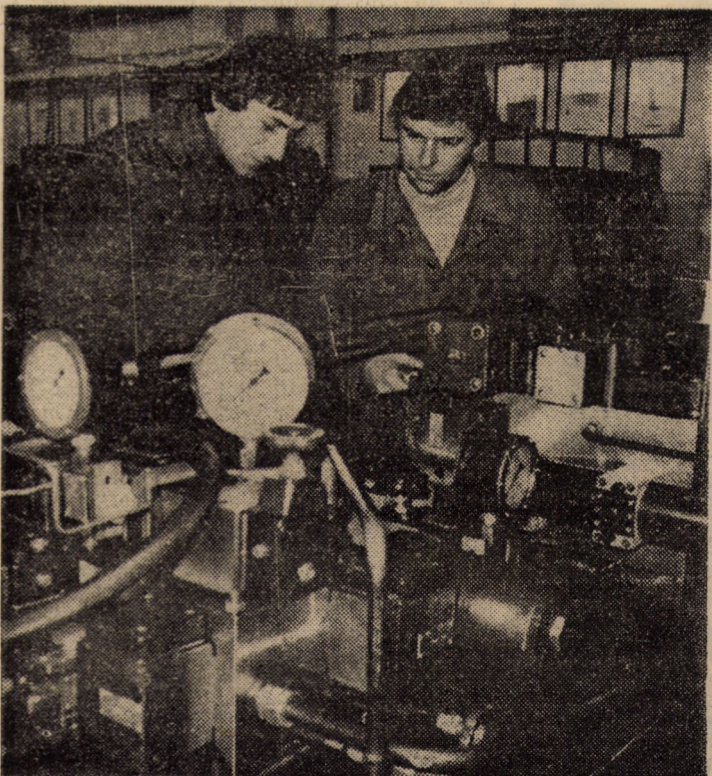
Tineri de la Fabrica de elemente hidropneumatice a întreprinderii „Balanta” Sibiu în fața unor panouri cu acționare hidraulică a mașinilor unelte
