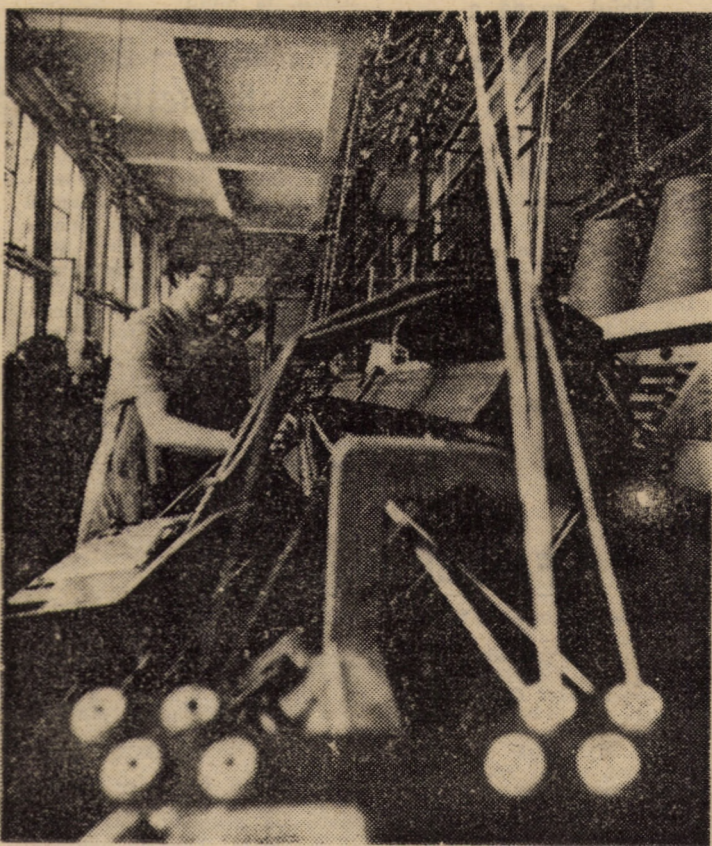
De la începutul acestui an, secția tricotație IV a întreprinderii „Drapelul roșu” din Sibiu a fost dotată cu un număr de 9 mașini rectilinii automate de tricotație, de tipul R 50, finețea 5 și 8, de producție românească. Noile utilaje de mare productivitate contribuie din plin la ridicarea calității produselor Foto: Fred NUSS
