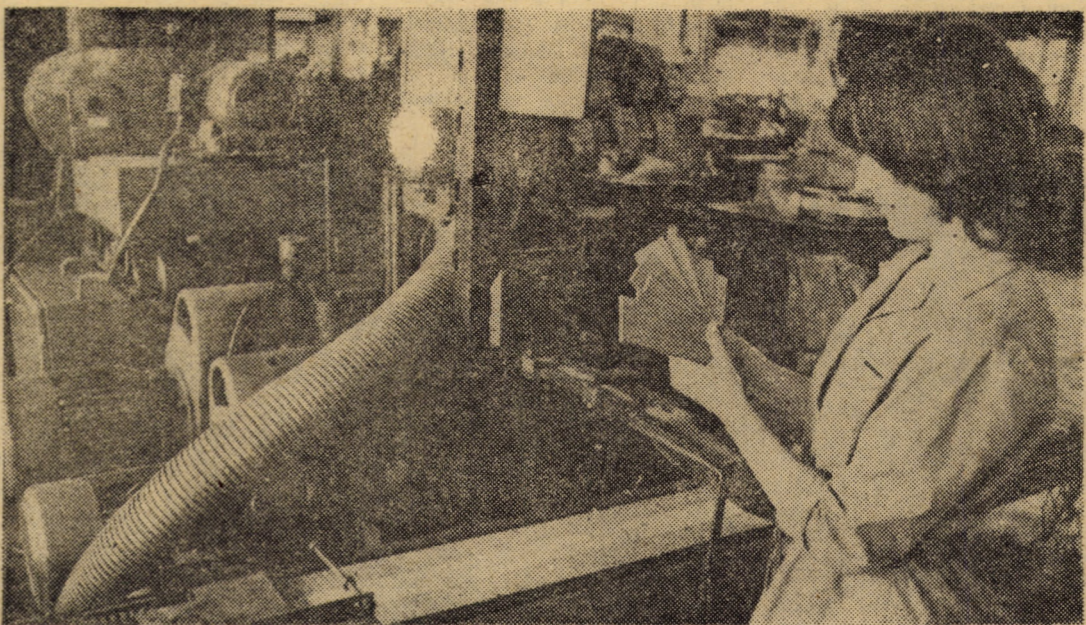
I.P.L. Sibiu, sectorul creioane: prezentăm în imagine operația de calibrare — pe toate fețele — a scindurelor, fază pregătitoare pentru linia automată de fabricat creioane
