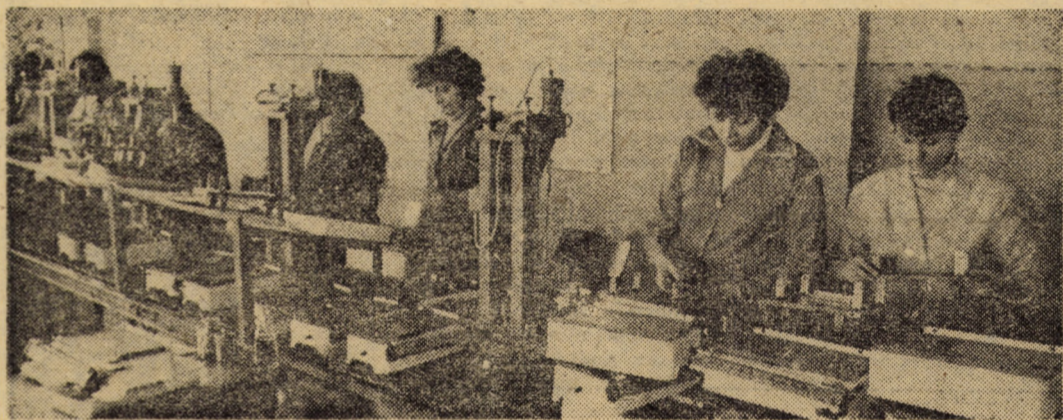
Vă redăm, în imaginea de față, linia de montaj final al balanțelor de 10 kg, pentru uz gospodăresc la întreprinderea „Balanta” Sibiu Foto: Fred NUSS
